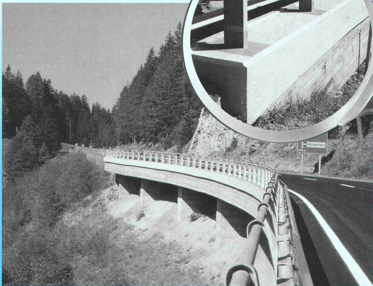
Lehnen-Viadukt, Tiefencastel
