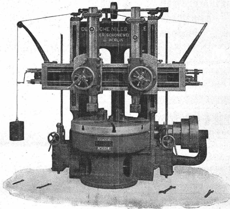
Karussell-Drehbank von 1000 mm Durchmesser.
