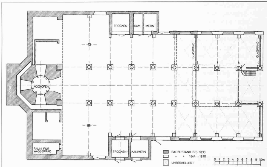
Grundriss der Sayner Hütte. Die Verwandtschaft mit dem Kirchenbau ist augenfällig
