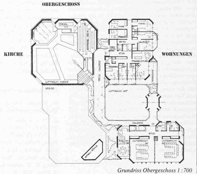
Grundriss Obergeschoss 1 : 700
