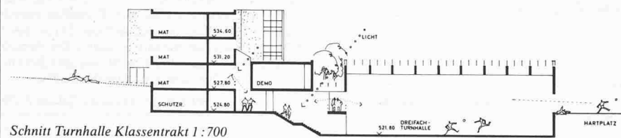
Schnitt Turnhalle Klassentrakt 1 : 700
