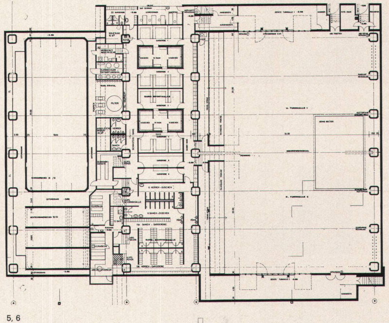
5 Grundriß Untergeschoß
