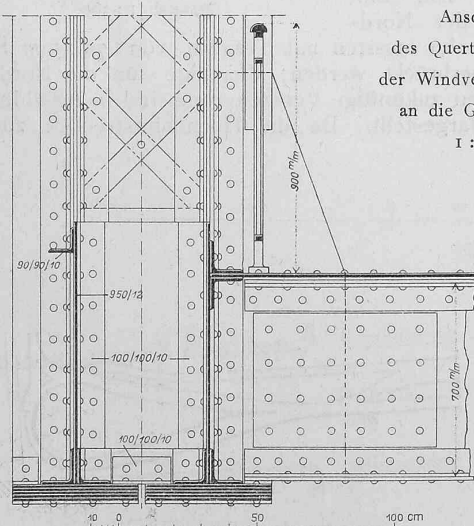
Abb. 10. Träger von 75,25 m Spannweite.
