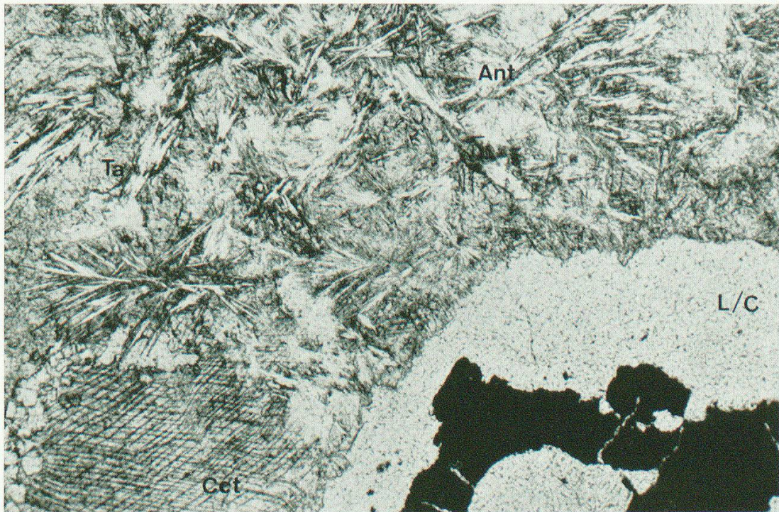
Fig. 3. Grüner Ophicalcit, der von Talk und Antigorit durchsetzt wird. D 1267, Koord. 768.27/151.82 (Westufer Marmorera-see). Rechts unten: Serpentin-komponente (Lizardit/Chrysotil mit Chromspinnellrelikt). Vergr. 51× mit gekreuzten Nicols.
