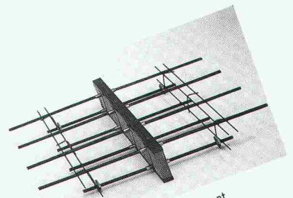
Kragplatten-Anschluss Standard-Element
