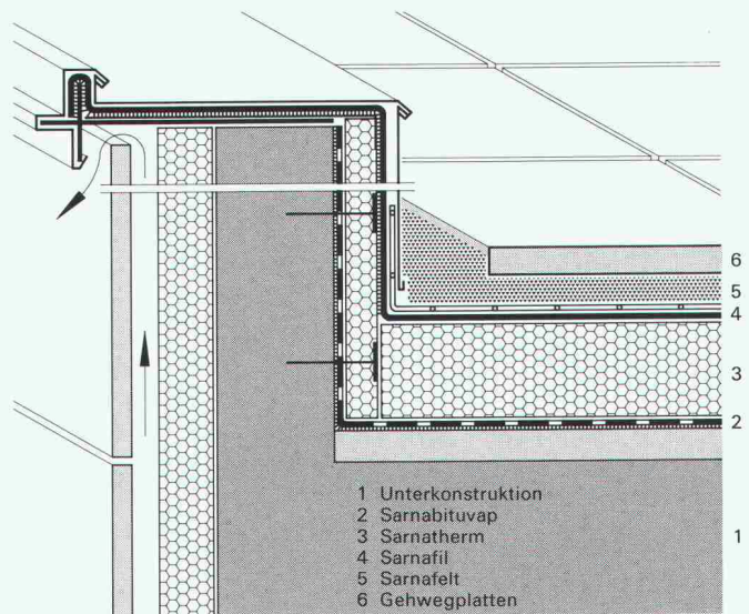
Dachrandabschluss für eine begehbare Sarnafil-Flachbedachung.
