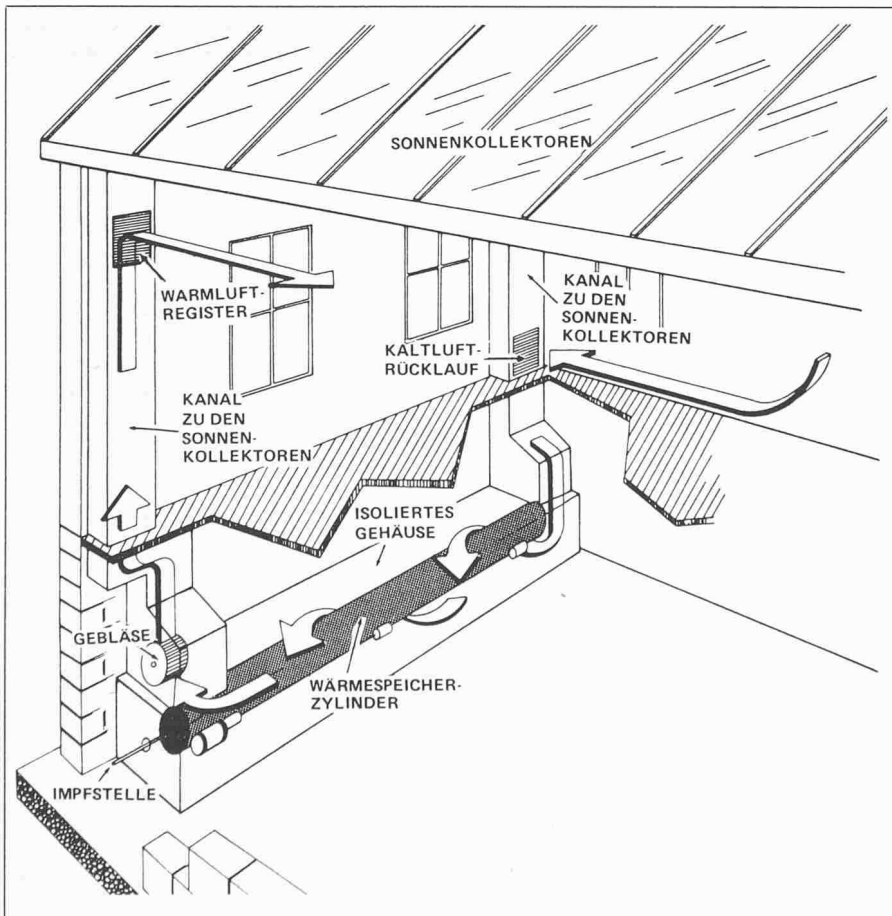
Eine der zahlreichen Verwendungsmöglichkeiten des Drehzylinder-Wärmespeichers ist der Einbau im Kellergeschoss eines Sonnenhauses. Bei Sonnenschein wird in den Sonnenkollektoren auf dem Dach erhitzte Luft dem Wärmespeicher zugeleitet, umspült dort den Drehzylinder und kühlt sich dabei ab. Die immer noch etwas warme Luft kann anschliessend zur Raumheizung dienen. Am Abend und an trüben Tagen schliessen sich Klappen in den Luftkanälen automatisch und trennen so die Sonnenkollektoren vom System ab. Das nunmehr von der Wärmezufuhr abgeschnittene Glaubersalz im Drehzylinder beginnt zu kristallisieren und gibt nach und nach die gespeicherte Latenzwärme ab. Die den Zylinder umspülende Luft erwärmt sich dabei und zirkuliert dann durch das Haus
