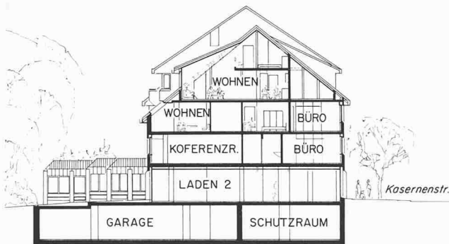
Schnitt 1:450
