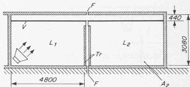
Bild 1. Vertikalschnitt durch einen Prüfstand zur Bestimmung der Längsdämmung von Deckenverkleidungen V Tr Trennwand von 180 mm Dicke und 4,75 m Breite mit einem R_w = 66 \text{ dB} , an Oberkante auf 100 mm Breite verjüngt F durchgehende Fuge zwischen den beiden Messräumen
