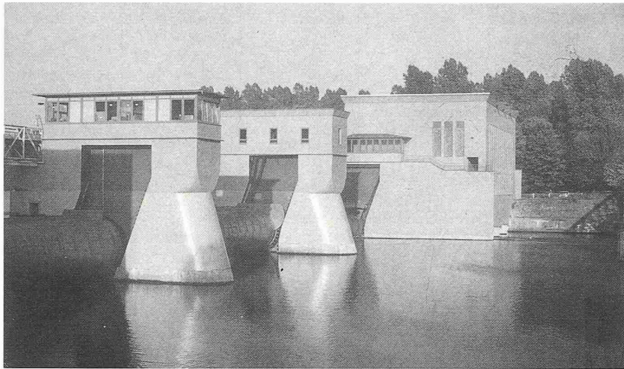
Bild 2. Wehranlage am Hengsteysee nach Sanierung der Wehrpfeiler mit Nassspritzmörtel - angeliefert als Werk trockenmörtel (Sager)
