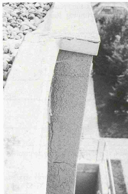
Bild 1. Die äussere Backsteinschale ist geknickt
