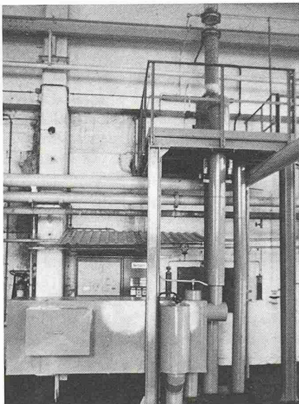
Bild 6. Schwefeläure-Hochkonzentrieranlage in Attisholz für die Chlortrocknung
