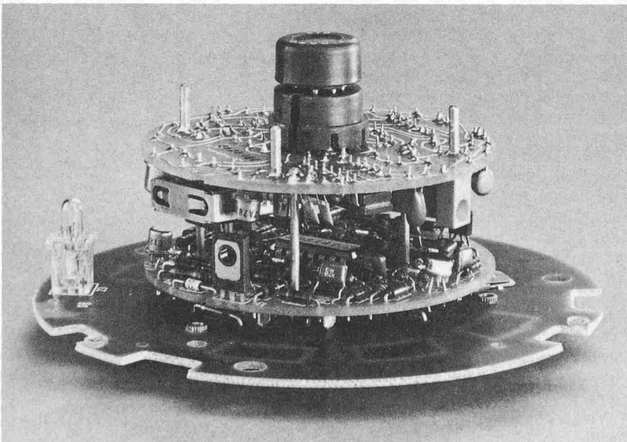
Bild 8. Cerberus-Gasmelder mit Halbleiter-Sensor, geöffnet. Der Halbleiter ist gut erkennbar; links aussen die Anzeigelampe, die bei Gasalarm blinkt. Die Empfindlichkeit des Melders kann je nach Bedürfnissen in vier Bereiche eingestellt werden
