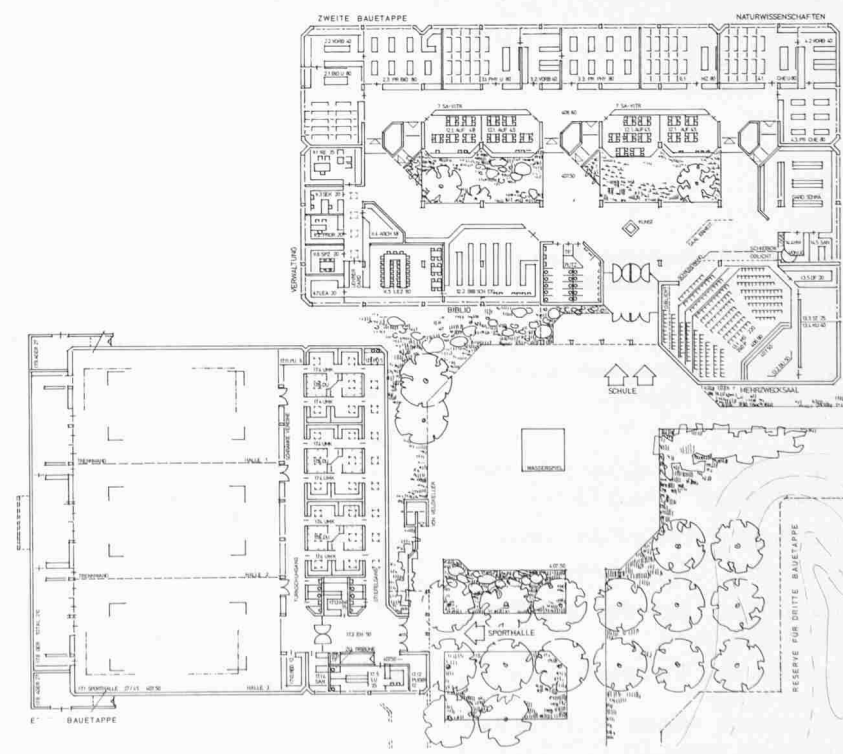
Grundriss Erdgeschoss 1:1000
