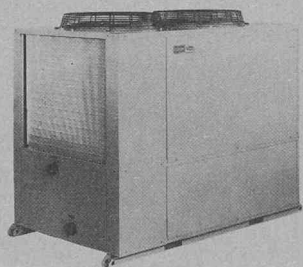
Hoval-Carrier-Wärmepumpe, Typ 30 AE/AQ. Kühlleistung 19–37 kW, Heizleistung 21–44 kW
