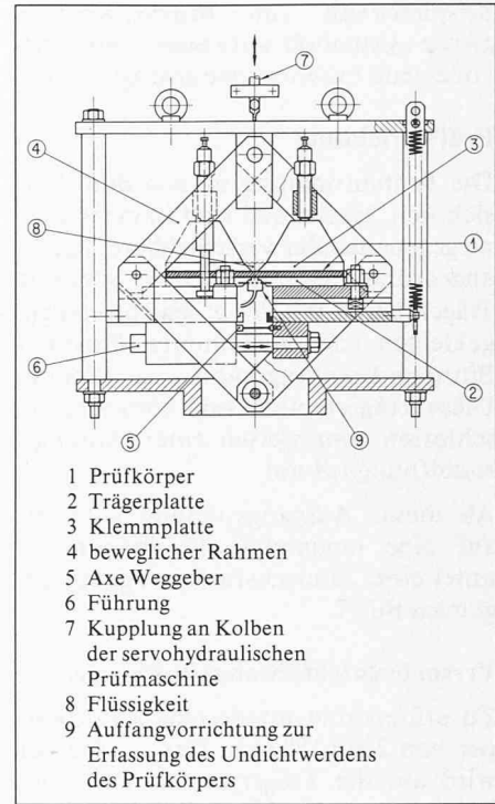
Bild 8. Einbau für Prüfung Nr. 11, Ermüdung in Prüfmaschine mit Klimakammer von -30\text{ }^{\circ}\text{C} bis +80\text{ }^{\circ}\text{C} gemäss Bild 9
