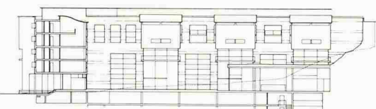
Schnitt G-G/Hof
