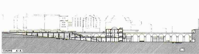
Coupe
