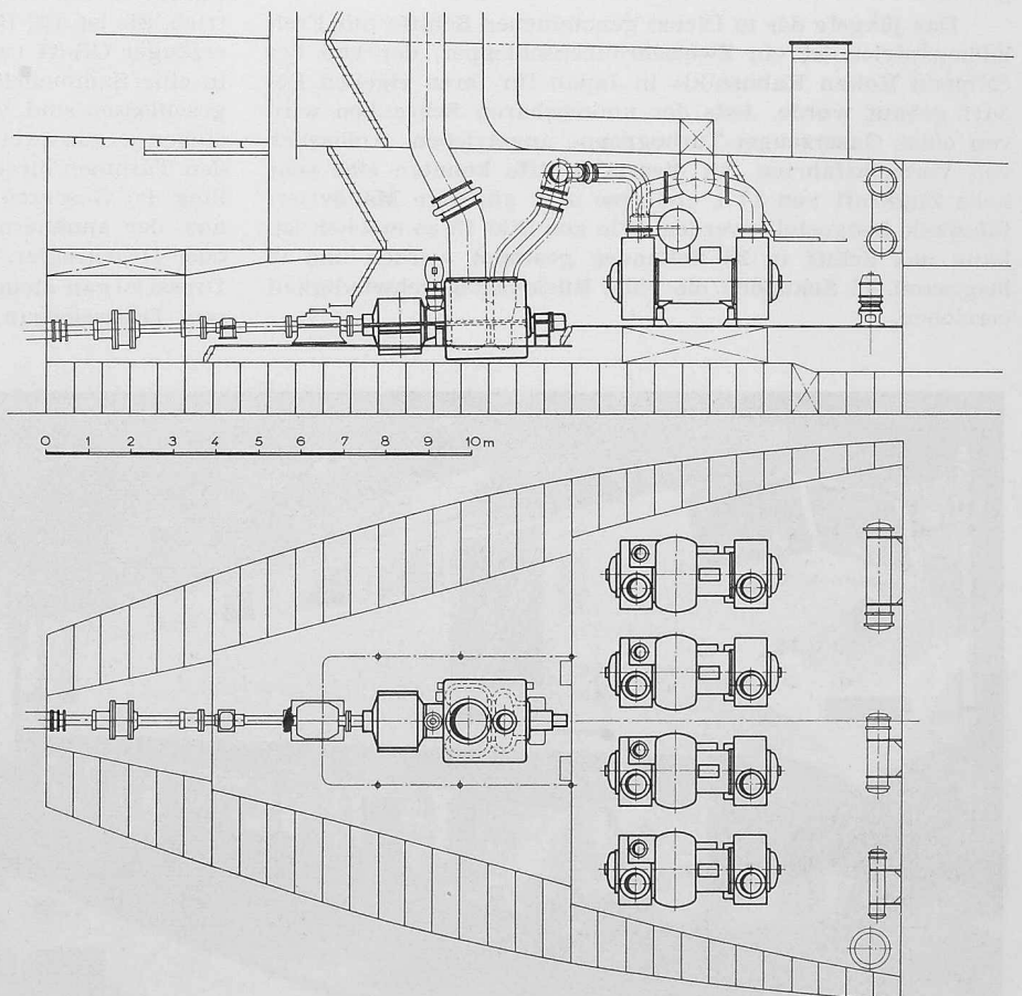
Bild 14. Anlage von 4000 PS der Firma Werkspoor auf einem Bananentransportschiff
