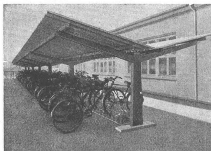
Fahrradhalter mit Ueberdachung, doppelseitige Ausführung. Typ HUD
