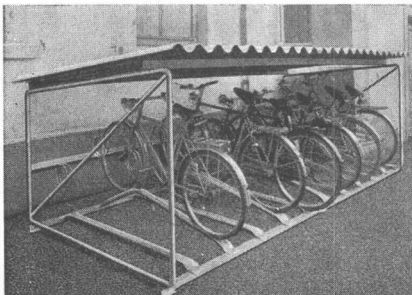
Serien-Fahrradklammern mit Ueberdachung und Einfahrkufen für hoch-tief-gestellte Fahrräder. Typ KU 10
