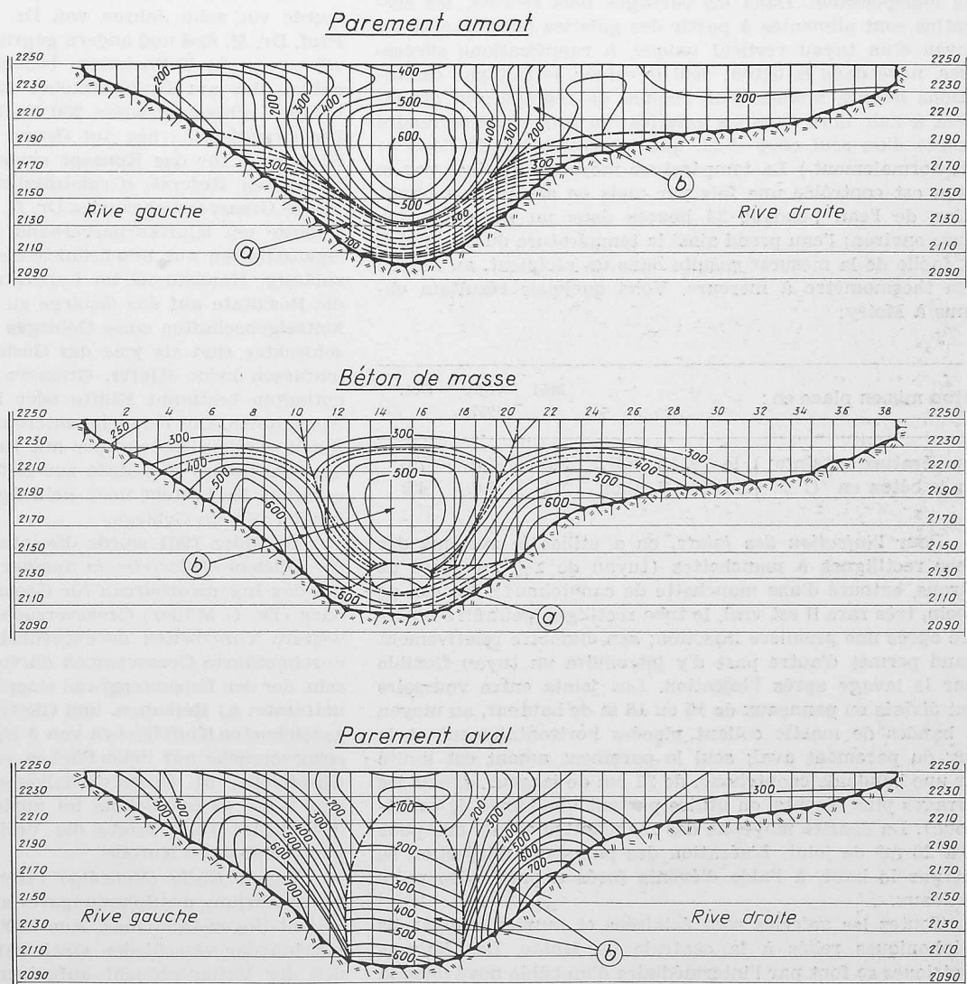
Fig. 10. Contraintes admissibles, en \text{t/m}^2 , pour fixer la résistance exigée du béton. a) Effet du poids propre seul. b) Effets cumulés du poids propre, de la poussée de l'eau et de la température
