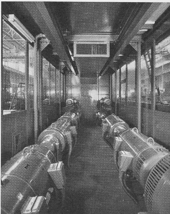
Bild 11. Leonard-Umformergruppen für eine grosse Werkzeugmaschine, eingebaut im staubfreien Raum unterhalb einer Blockanlage
