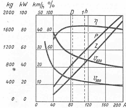
Abb. 8. Charakteristische Kurven des Motors. P Motorleistung in kW am Triebgrad. Z Zugkraft in kg am Triebgradumfang. η Totaler Wirkungsgrad (einschl. Getriebe). v Fahrgeschwindigkeit.
