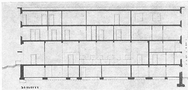
IV. Preis (1000 Fr.), Entwurf Nr. 8. Verfasser Albert Schellenberg, Architekt, Kreuzlingen. Lageplan 1 : 2000, Grundrisse und Schnitte 1 : 400, Ansicht von N. O.
