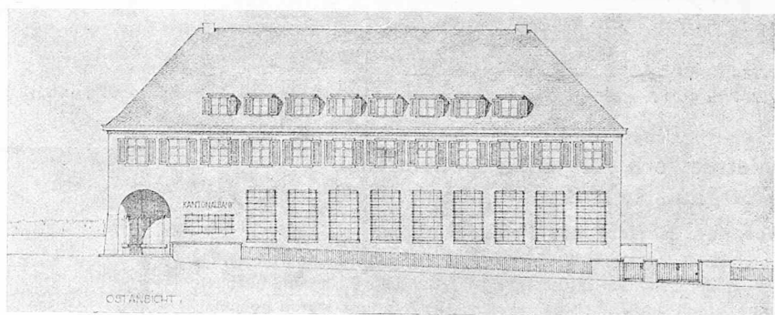
Ostfassade 1 : 400.
