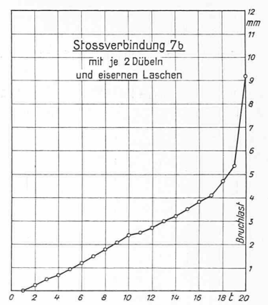
Abb. 12. Gemessene Verschiebungen: 7 A volle Linie linke, gestrichelte rechte Stosshälfte. 7 B Verschiebungen auf je eine der Stosshälften bezogen (halbe Fugenweite).
