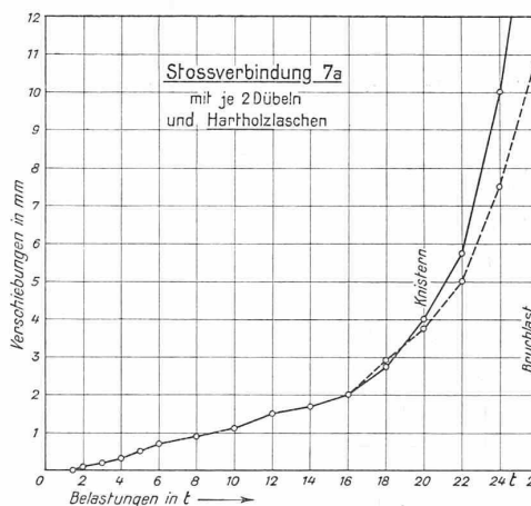
Abb. 12. Gemessene Verschiebungen: 7 A volle Linie linke, gestrichelte rechte Stosshälfte. 7 B Verschiebungen auf je eine der Stosshälften bezogen (halbe Fugenweite).
