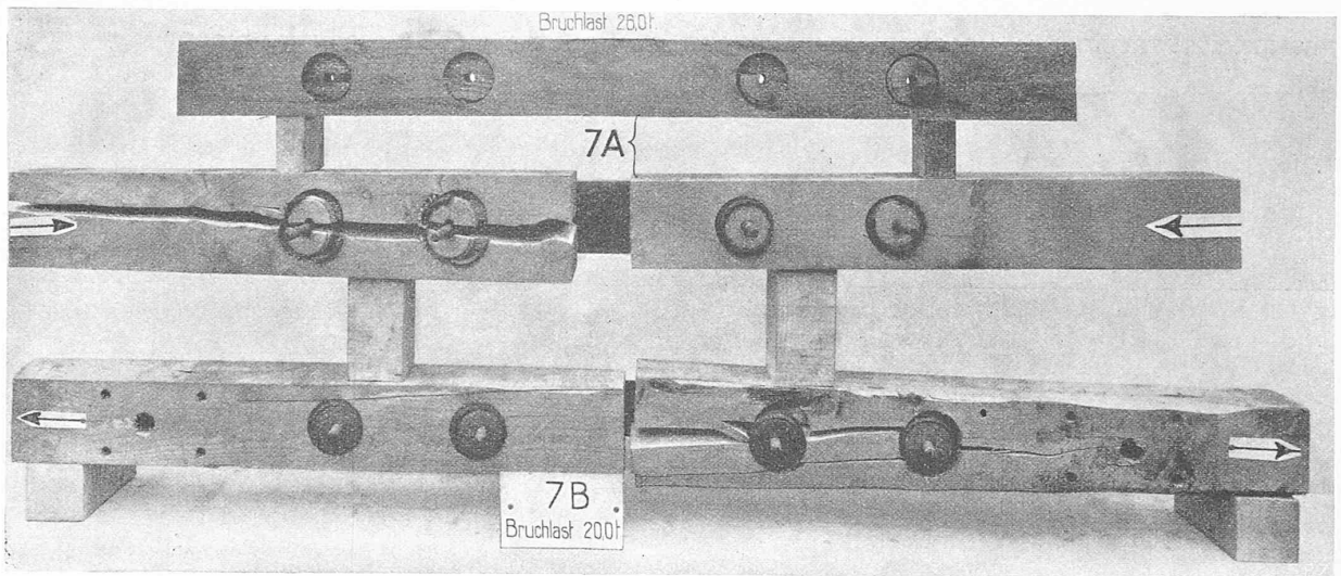
Abb. 11. Probekörper Nr. 7 A mit Hartholzlaschen, Nr. 7 B mit Eisenlaschen.
