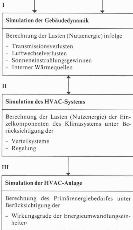
Rechenphasen bei der Ermittlung des Energiebedarfes von klimatisierten Gebäuden
