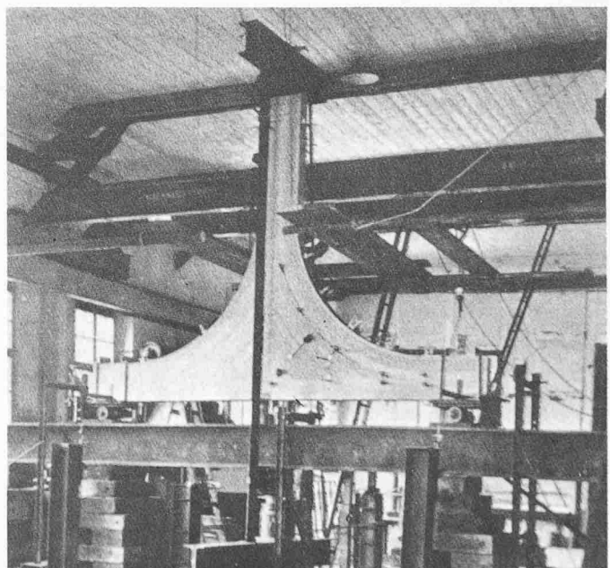
Bild 18. Versuche an einstielligen Perronbindern 1944. Kreisdirektion II der SBB in Zusammenwirken mit der EMPA. Der untersuchte Typ wurde in mehreren SBB-Bahnhöfen ausgeführt, so u. a. in Däniken [22]
