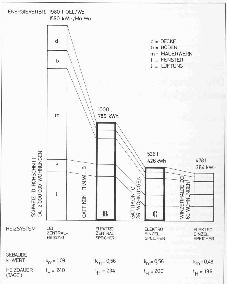
Bild 6. Energieverbrauch der einzelnen Bauglieder einer Durchschnittswohnung von 3,3 Zimmern bei verschiedenen Heizsystemen. Öl- und Elektrozentralheizung; Kollektivheizungen; Elektroeinzelpeicher; Individualheizung
