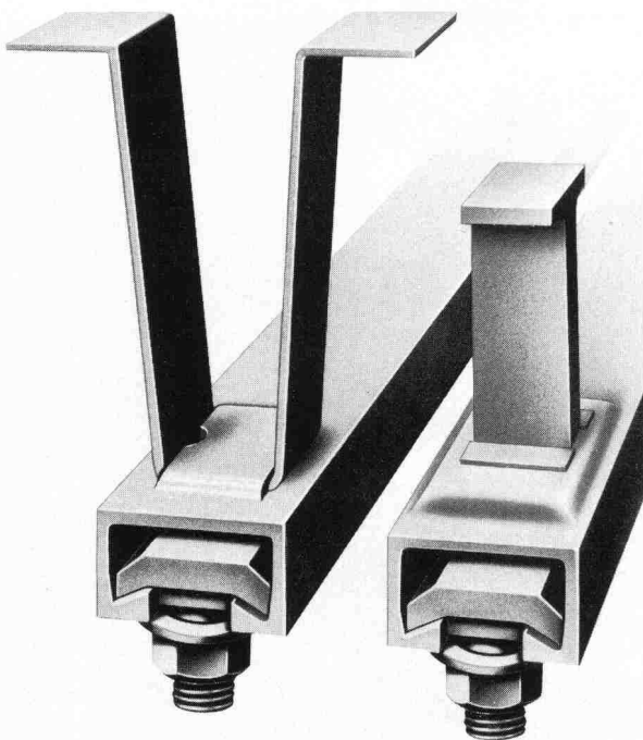
HSB-HALFENEISEN mit losen Verankerungsbügeln max. Belastung 35-120 kN/m
