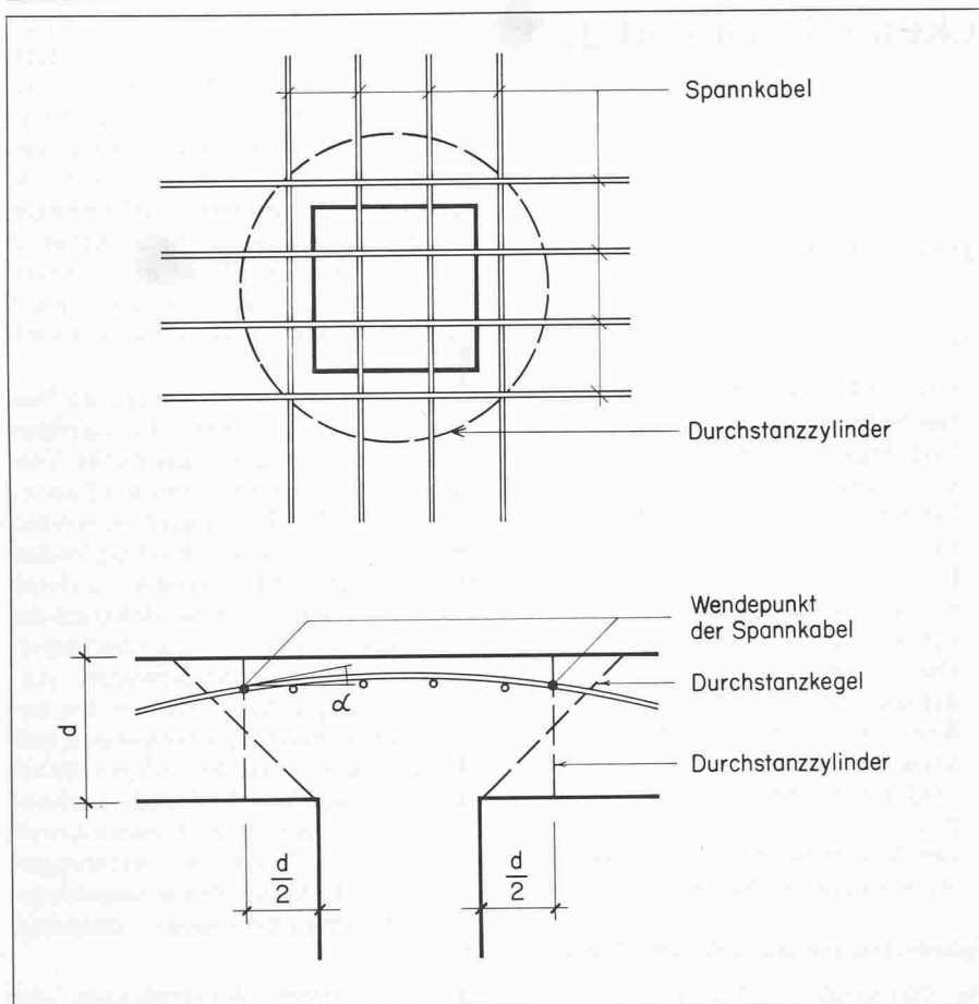
Bild 2. Kabelverlauf im Bereich des Durchstanzzylinders um eine innere Stütze (schlaffe Bewehrung nicht eingezeichnet)
