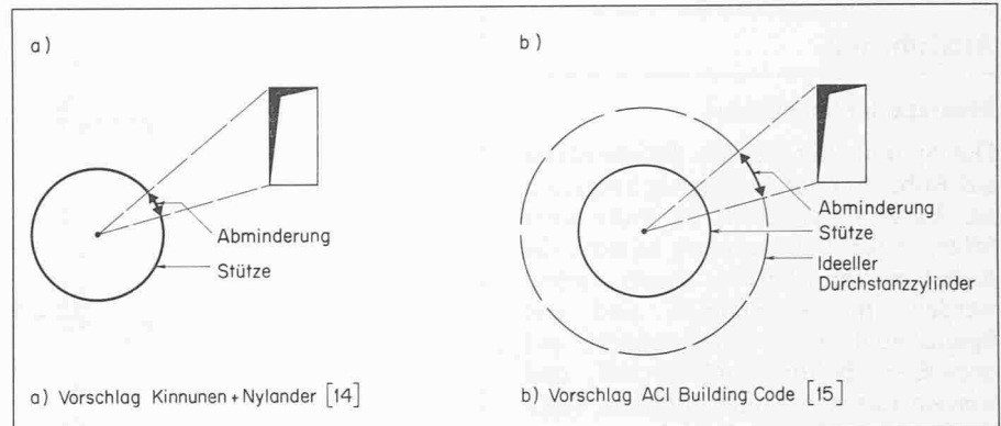
Bild 6. Abminderung des Umfanges des Durchstanzzylinders infolge Aussparungen im Stützenbereich (Bereich 3)
