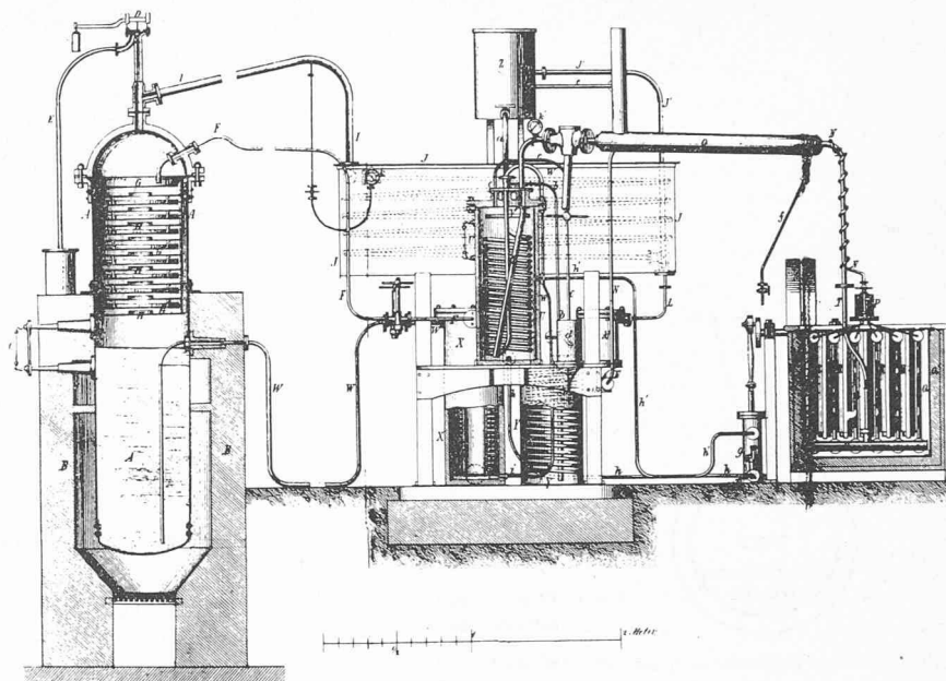
Bild 3. Carrés Apparat zur kontinuierlichen Eisfabrikation
