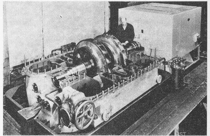
Bild 6. Zweistufiges Radialgebläse mit Vorrotationsregelung beider Stufen. Max. Fördermenge 110 000 m 3 /h, Förderdruck 1,55 bar abs., Antriebsleistung 2250 kW. Vorne links ist der Ansaugraum sichtbar mit den drehbaren Klappen für die Vorrotationsregelung. Nach dem Austritt aus dem ersten Rad strömt die Luft in den radialen Diffusor und wird dann um 180° umgelenkt für den Eintritt in das zweite Rad (Gebrüder Sulzer Aktiengesellschaft, Winterthur)
