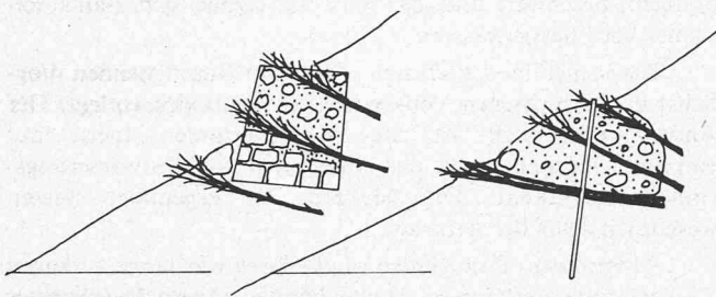
Bild 5. Begrünter Drahtschotterkörper, links aus verschweissten Stahlgittern, rechts aus elastischerem Drahtnetz, jeweils mit Buschlagen (Schema)
