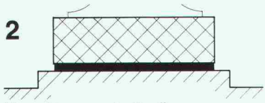
2 Maschinensockelisolierung
