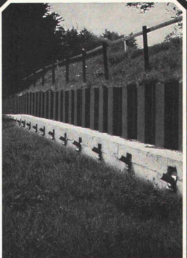
Rutschsanierung Hüntwangen
