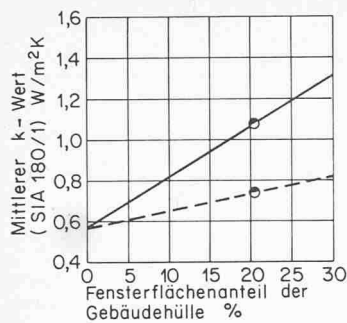
Bild 2. Einfluss des Fensteranteils der Gebäudehülle auf den mittleren k -Wert der Gebäudehülle des Fabrikationsgebäudes. Definition und Berechnung von \bar{k} nach SIA 180/1
