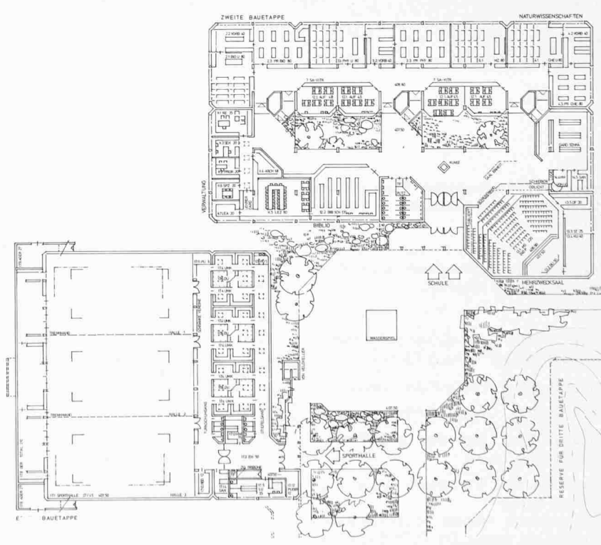
Grundriss Erdgeschoss 1:1000
