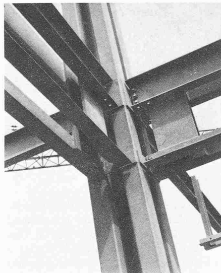
Detailansichten Stützenanschlüsse
