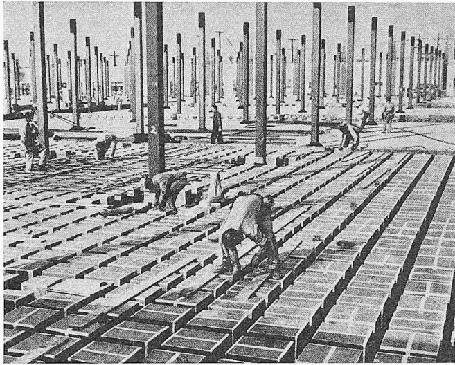
Fig. 3. On dispose les hourdis en carton
