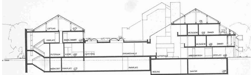
SCHNITT C-C
