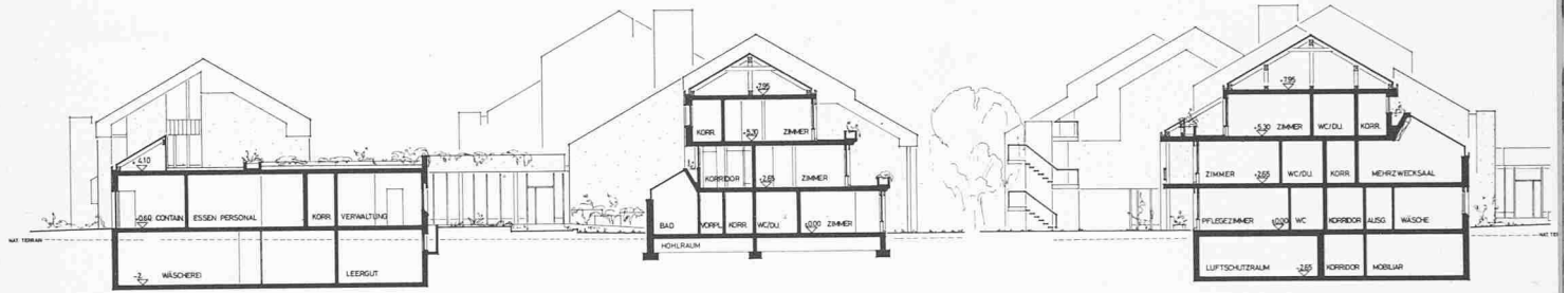
SCHNITT D-D
