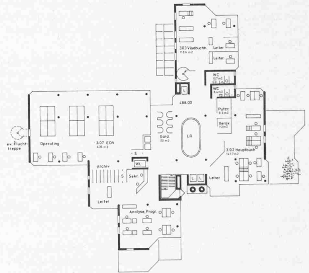
Oben: Grundriss 3. Obergeschoss 1:700 Links: Grundriss Erdgeschoss 1:700 Unten: Schnitt A-A 1:700, Parkgarage
