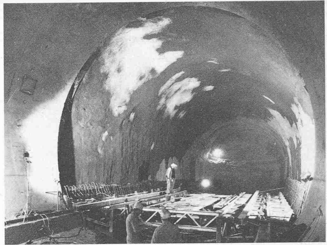
Bild 18. Vollaussbruch einer Etappe und Betonieren des Sohlgewölbes
