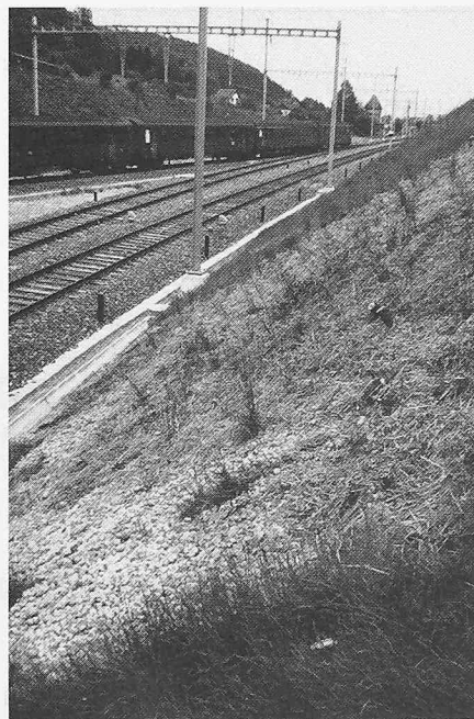
Den wiederhergestellten Rutschflächen fehlt ein Erosionsschutz. Deshalb wurden sie mit langhalmigem Stroh ausgelegt, angesät und leicht mit Bitumen fixiert
