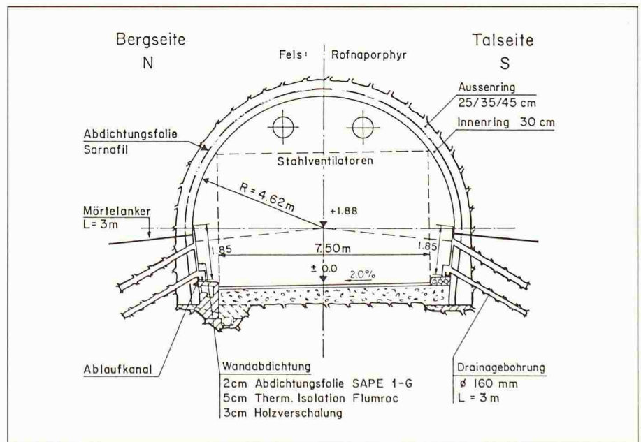
Bild 2. Die Sanierung des Rofla-Tunnels der Nationalstrasse N13, u.a. mit thermischer Isolierschicht zum Vermeiden von Eisbildung (R. Mettler)
