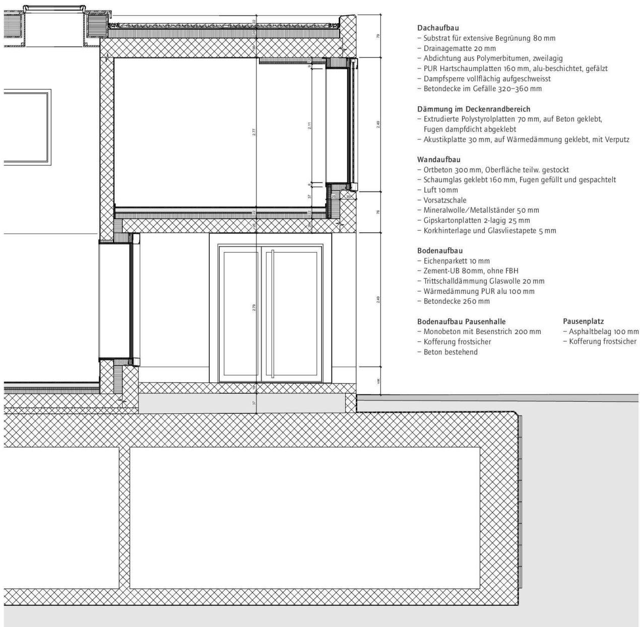
Detailschnitt
