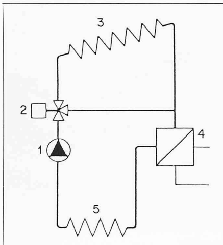
Kombination Luftregister/Erdkollektor 1 Umwälzpumpe 2 Verteilventil 3 Luftregister Carport 4 Verdampfer, Wärmepumpe 5 Erdkollektor
