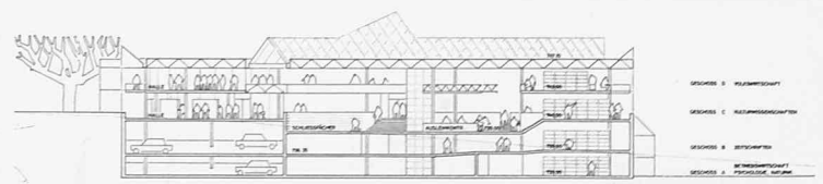
Schnitt C-C 1:900
