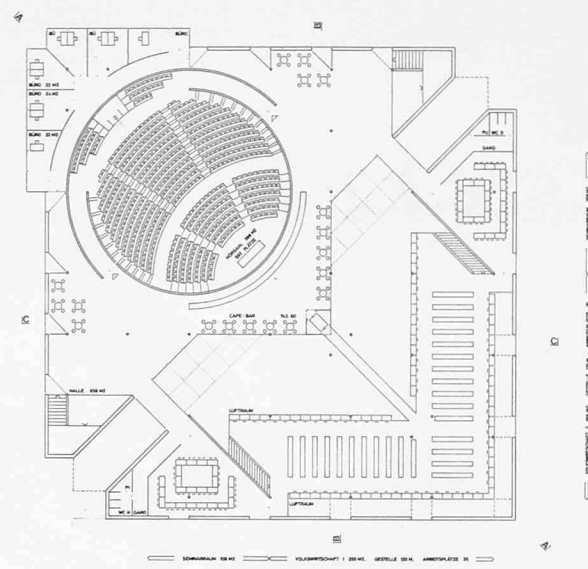
Geschoss D, 743.60, 1:900
